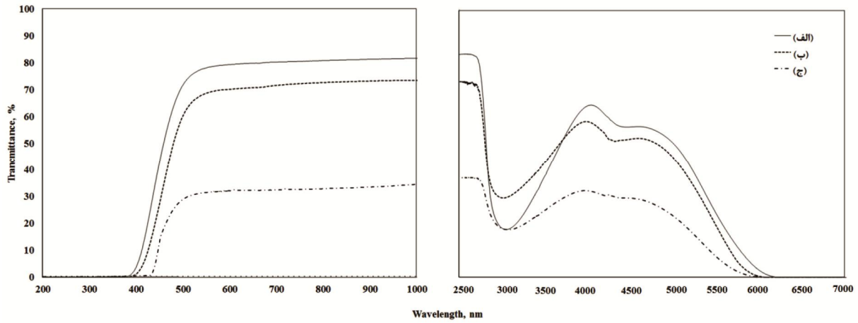
شکل ۶- نمودارهای عبورپذیری مربوط به شیشه‌های 50\text{GeO}_2\text{-}(50-x)\text{PbO}\text{-}x\text{CaO} در حضور: (الف) صفر، (ب) 10^\circ و (ج) 20^\circ درصد مولی اکسید کلسیم (با ضخامت سه میلی‌متر)
