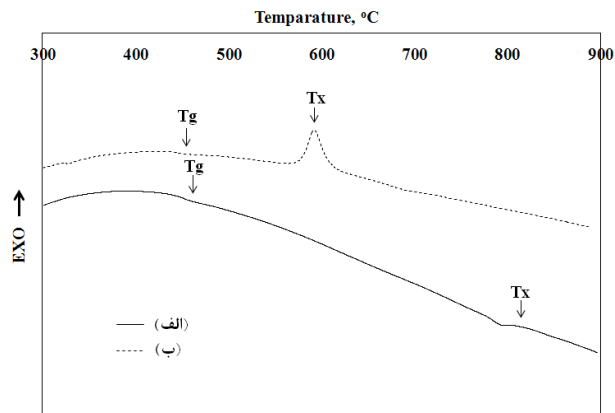
شکل ۳- نمودارهای آنالیز حرارتی مربوط به شیشه‌های 5^\circ\text{GeO}_2-(5^\circ-x)\text{PbO}-x\text{CaO} در حضور: الف) صفر و ب) ۱۰ درصد مولی اکسید کلسیم
