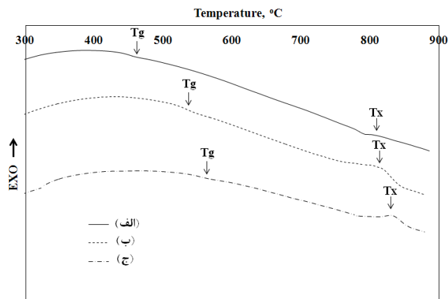
شکل ۴- نمودارهای آنالیز حرارتی مربوط به شیشه‌های 5^\circ\text{GeO}_2-(5^\circ-x)\text{PbO}-x\text{SrO} در حضور: الف) صفر، ب) ۱۰ و ج) ۲۰ درصد مولی اکسید استرانسیم
