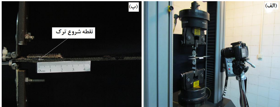
شکل ۳- الف) نمایی از دستگاه کشش در حین آزمایش برش بین لایه‌ای و ب) نحوه قرار گرفتن نمونه در بین فک‌های دستگاه
