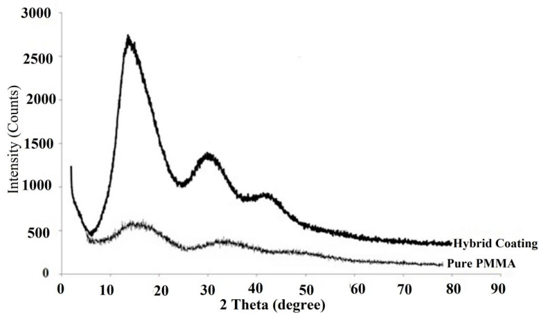
شکل ۱- الگوی پراش پرتو ایکس پوشش بهینه
