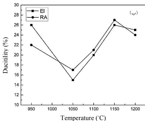
شکل ۷- الف) تغییرات تنش حداکثر با دما و ب) تغییرات داکتیلیته با دما برای آلیاژ Haynes 25
