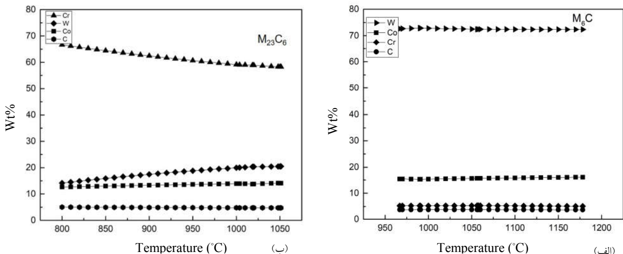
شکل ۴- ترکیب شیمیایی کاربیدهای موجود در آلیاژ Haynes 25 و تغییرات آن با دما (الف) M_{23}C_6 و (ب) M_6C ، به دست آمده از نرم افزار JMat pro
