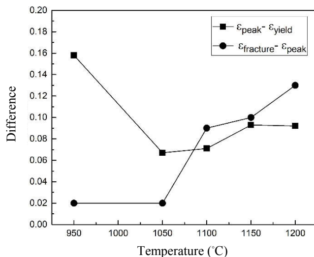
شکل ۸- بررسی اختلاف بین کرنش نقطه حداکثر و تسلیم ( \epsilon_{\text{yield}} - \epsilon_{\text{peak}} ) و نقطه شکست و حداکثر ( \epsilon_{\text{fracture}} - \epsilon_{\text{peak}} )
