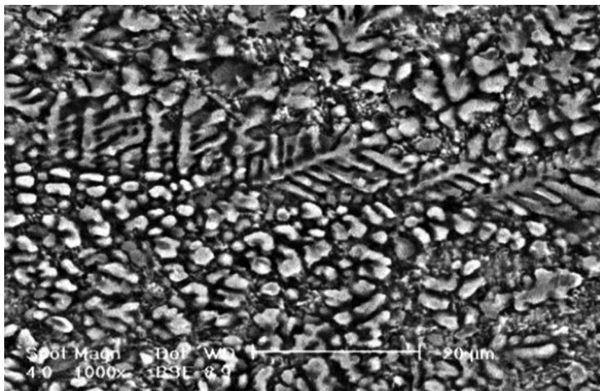
شکل ۴- تصویر میکروسکوپی الکترونی روبشی از نمونه آلیاژسازی شده با کروم و نیتروژن (P4)
