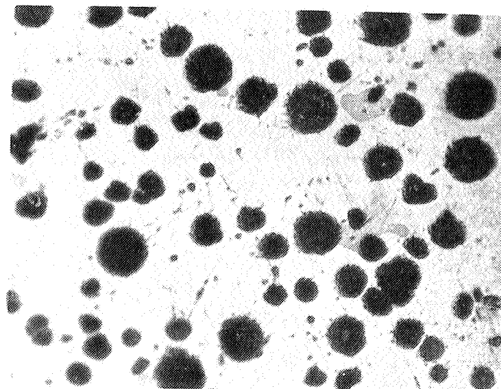
شکل ۸ - ساختار میکروسکوپی آلیاژی با ۱/۵ درصد مس بحالت ریختگی محلول طاهر کننده معرف نشده و بزرگ نمائی ۱۰۰ برابر است
