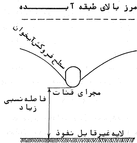
شکل ۳ - نمایش شماتیک مجرای قنات
