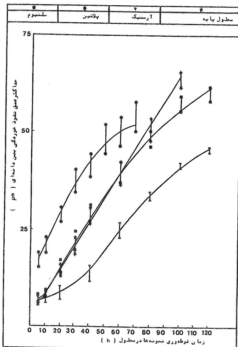
شکل ۱۱ : تأثیر زمان غوطه‌وری بر حداکثر عمق نفوذ خوردگی بین داده‌ای در محلول پایه و محلول پایه حاوی ۲۵ ppm از سموم کاتدی مختلف .
