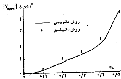
ج - حداکثر نیروی برشی
