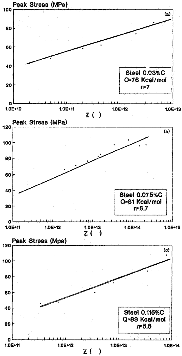
شکل ۸ - رابطه بین پارامتر زنو - هولمن با تنش پیک . (a) فولاد B (b) فولاد C (c) فولاد D
