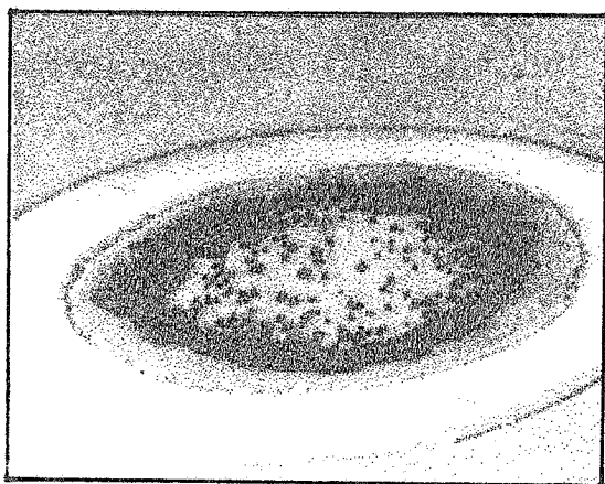
شکل ۶- تصویر میکروسکوپی الکترونی از چگونگی توزیع کریستالهای الماس تشکیل شده بر روی زیر لایه فولاد زنگ نزن آستنیتی در دمای بالا
