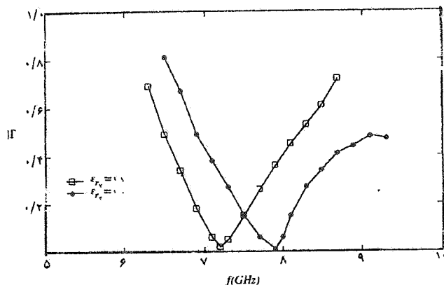
شکل ۶- تأثیر روبنا بر روی ضریب انعکاس آنتن مثال (۳)، a=1\text{cm} ، d_s=0/3\text{cm} ، w_a=0/03\text{cm} ، d_a=1/0\text{cm} ، b=1/4\text{cm} ، d_1=0/317\text{cm} ، \epsilon_{rf}=6/15 ، \epsilon_{r1}=2/33 ، w_f=0/2773\text{cm} ، d_f=0/1905\text{cm} ، d_v=0/2\text{cm}
