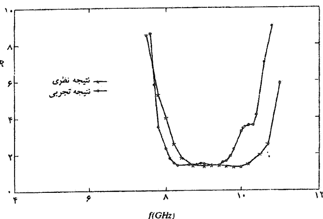
شکل ۷- نتیجه تجربی و نظری برای VSWR آنتن مثال (۴)، w_a=0/04\text{cm} ، d_a=0/75\text{cm} ، b=1/1\text{cm} ، a=0/7\text{cm} ، d_1=0/317\text{cm} ، \epsilon_{rf}=6/15 ، w_f=0/09\text{cm} ، d_s=0/11\text{cm} ، d_f=0/0614\text{cm}
