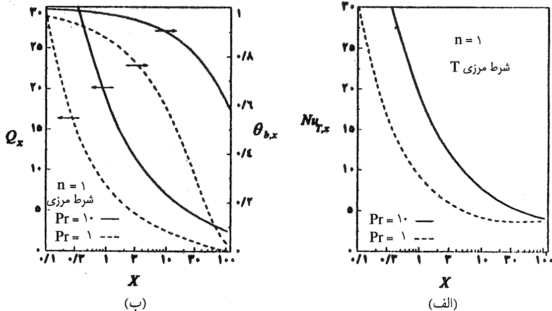
شکل ۱۰- مشخصات گرمایی بر حسب X برای شرط مرزی T و اعداد پراتل متفاوت Re = 500
