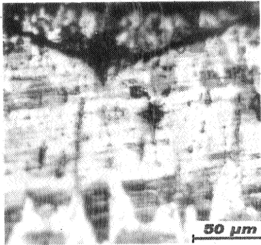
شکل ۷- ریزساختار لایه بررونایز شده در دمای ۹۵۰ °C به مدت ۴ ساعت همراه با ترک ایجاد شده در اثر ایندنتور دستگاه ریزسختی سنج
