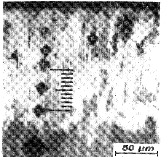
شکل ۶- ریزساختار لایه بررونایز شده در دمای ۹۵۰ °C به مدت ۴ ساعت
