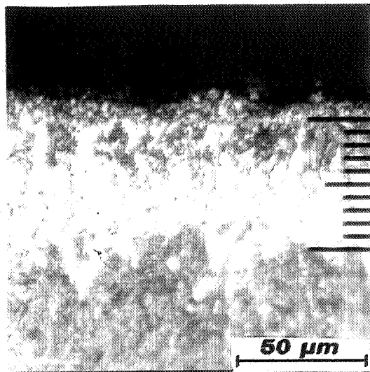
شکل ۱۰- ریزساختار لایه بروسلیکونایز ایجاد شده از مخلوط ۸۵٪ پودر برونایز + ۱۵٪ پودر سیلیکونایز (ترکیب ردیف ۱۱ جدول ۱)
