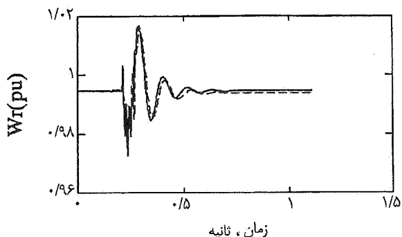
شکل ۱۳- تغییرات سرعت موتورها در سیستم اول در حالت اتصال کوتاه ( N_L=60 , CSVC--, OSVC_, RSVC_)
