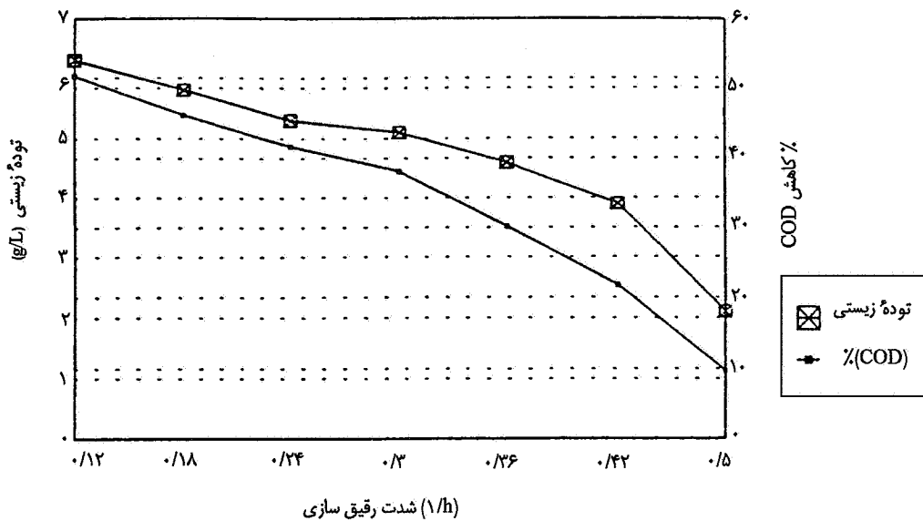
شکل ۸- تغییرات توده زیستی و درصد کاهش XO\Delta با شدت رقیق سازی. دمای 34^{\circ}C ، شدت هوادهی 27.7m ، دور همزن 0.08 \pi. \mu ، pH اولیه محیط کشت 3/5
