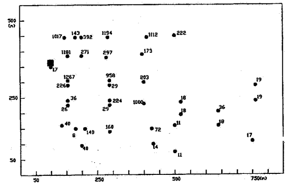
شکل ۱- مراکز بار و محل تغذیه اصلی در یک کارخانه شیمیایی در شکل نمایش داده شده است
