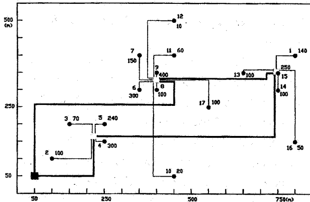
شکل ۸- طرح زیر بهینه نمونه مورد مطالعه شماره (۲) با سه پست فرعی
