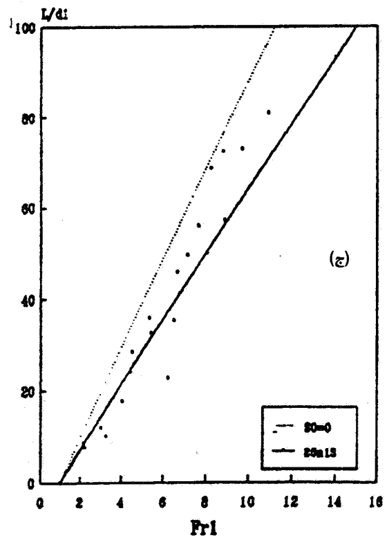
شکل ۴- مقادیر L/d_1 نسبت به Fr_1 برای پله با ارتفاع ۲۵ میلیمتر در شیب معکوس الف) ۰/۵ درصد (ب) ۱ درصد (ج) ۱/۳ درصد (د) ۲ درصد
