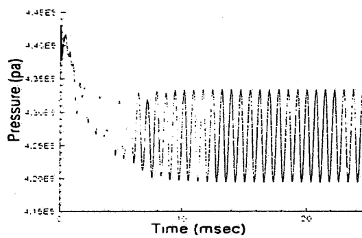
الف - فشار در نقطه ۲
