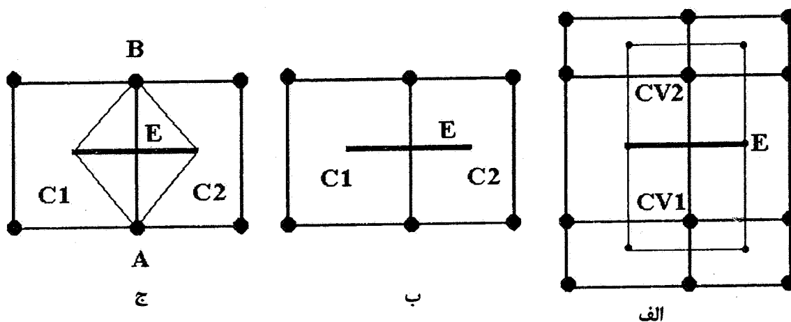
شکل ۳- درونیابی شار لزوج
