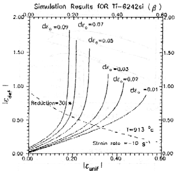
شکل ۹- کرنش در ناحیه معیوب بر حسب کرنش در ناحیه غیر معیوب برای آلیاژ (\beta) Ti 6242 Si در T=913^{\circ}\text{C} و \dot{\epsilon}_0 = 10\text{s}^{-1} برای d\epsilon_0 های نشان داده شده
