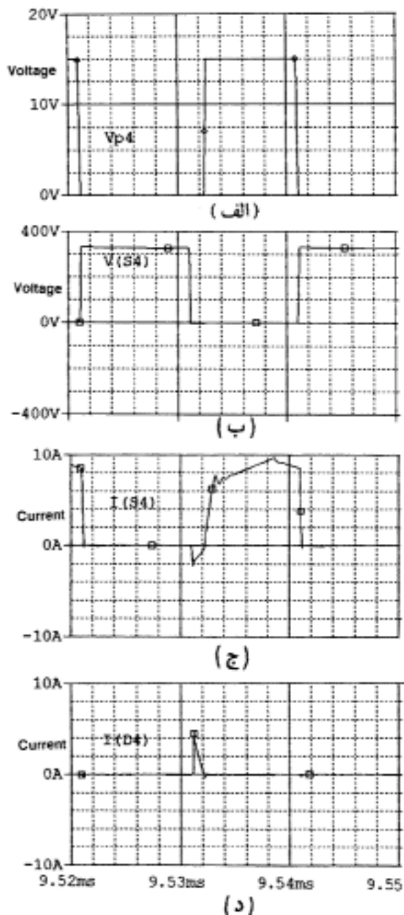
شکل ۶- شکل موجهای شاخه پس فاز میدل ZVS با سلف نشی الف- پالس درایو گیت سورس، ب- ولتاژ درین سورس ج- جریان کلید پسفاز، د- جریان دیود موازی معکوس کلید
