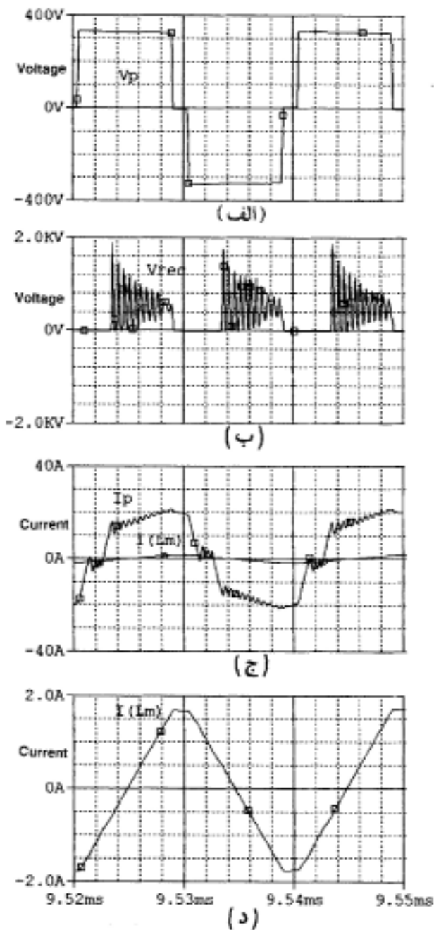
شکل ۷- میدل ZVS با سلف مغناطیس کنندگی الف- ولتاژ اولیه ب- ولتاژ ثانویه: ج- جریان اولیه و جریان سلف مغناطیس کنندگی د- جریان سلف مغناطیس کنندگی (شکل بزرگ شده)
