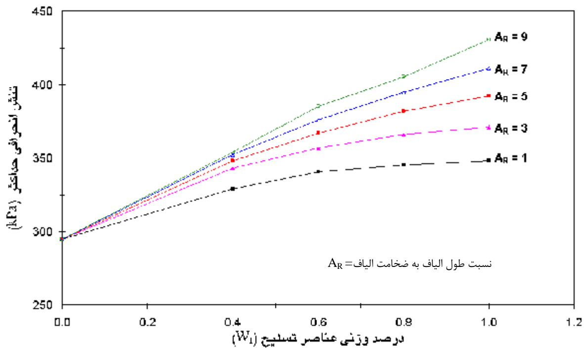
شکل ۷- تغییرات تنش انحرافی حداکثر بر حسب درصد وزنی عناصر تسلیح W_f و نسبت اضلاع عناصر A_R در آزمایش سهمجوری CD ( s'_c = 100 kPa)
