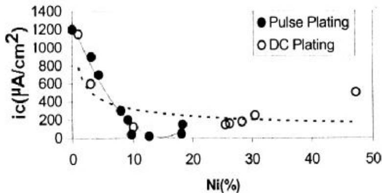
شکل ۷- تاثیر درصد نیکل در چگالی جریان خوردگی پوششهای آلیاژی روی- نیکل حاصل از آبکاری الکتریکی مستقیم و منقطع
