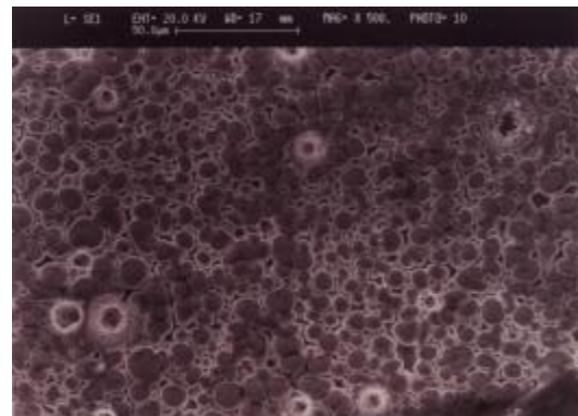
شکل ۲- تصویر SEM از سطح پوشش حاصل از روش مستقیم با ترکیب آلیاژی Zn=۰/۵۲/۸ و Ni=۰/۴۷/۲ و شرایط آبکاری I = 11 \text{ A/dm}^2 ; T = 60^\circ \text{C} ; \text{pH} = 2
