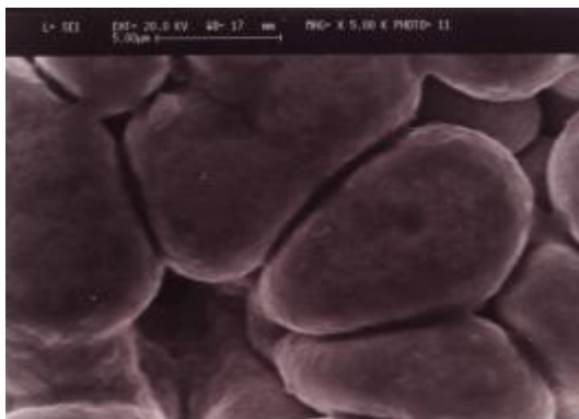
شکل ۲- تصویر SEM از سطح پوشش حاصل از روش مستقیم با ترکیب آلیاژی Zn=۰/۵۲/۸ و Ni=۰/۴۷/۲ و شرایط آبکاری I = 11 \text{ A/dm}^2 ; T = 60^\circ \text{C} ; \text{pH} = 2
