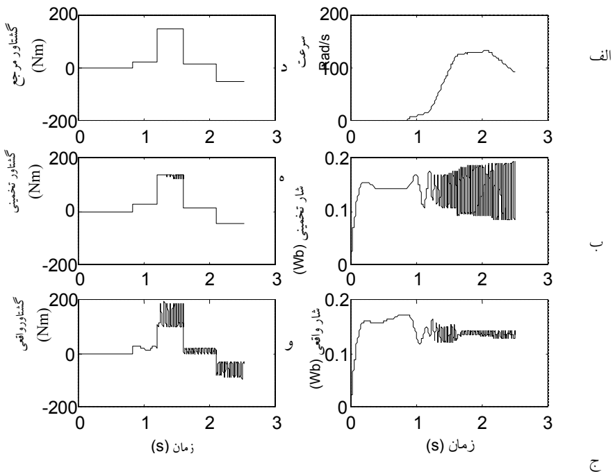
شکل ۷. عملکرد سیستم با استفاده از LPIF برای حل مشکل dc offset الف- سرعت ب- شار تخمینی ج- شار واقعی د- گشتاور مرجع ه- گشتاور تخمینی و- گشتاور واقعی
