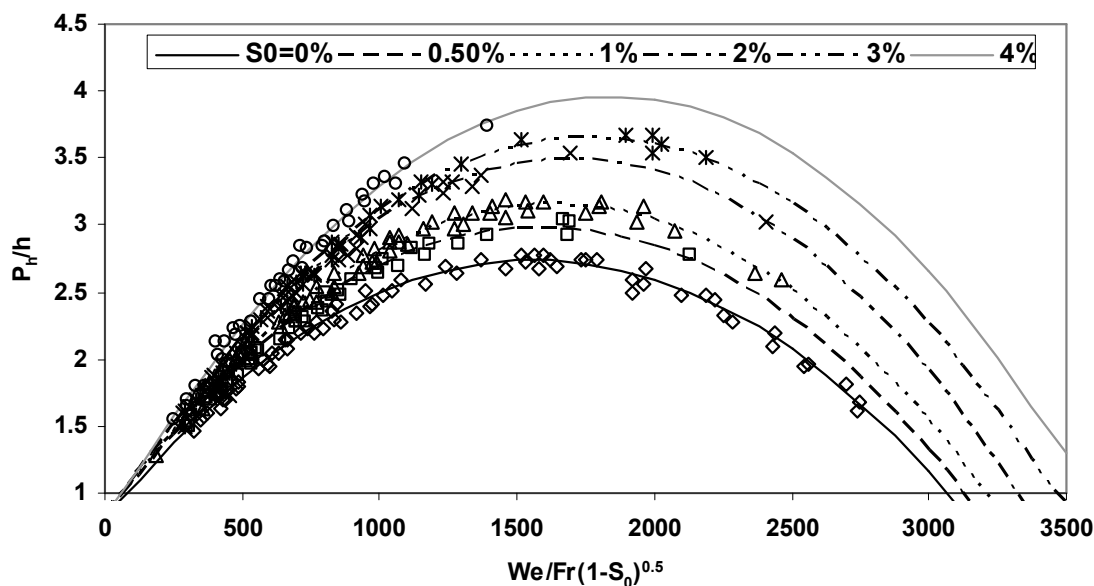
شکل ۱۶- تغییرات فشار متوسط بر حسب wfs در شبیه‌های مختلف
