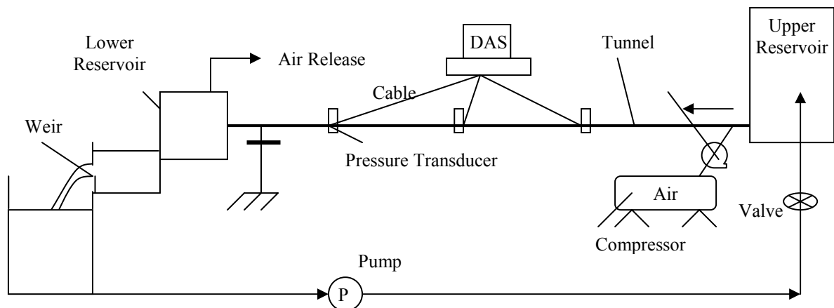
شکل ۱- شمای کلی بخشهای مختلف مدل آزمایشگاهی
