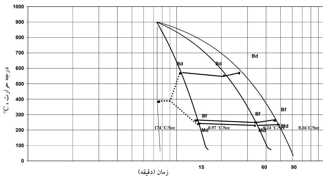
شکل ۳- نمودار CCCT فولاد NiCrMoV در حالت یک مرحله کرنش روی آستنیت اولیه در دمای 900^{\circ}\text{C} ، با نرخ کرنش 0.1/\text{s} و کرنش 0.92\% ، به معنای بینایت و M، به معنای مارتنزیت است نقاط نقطه چین، نقاط آزمایش نشده احتمالی را نشان می‌دهد
