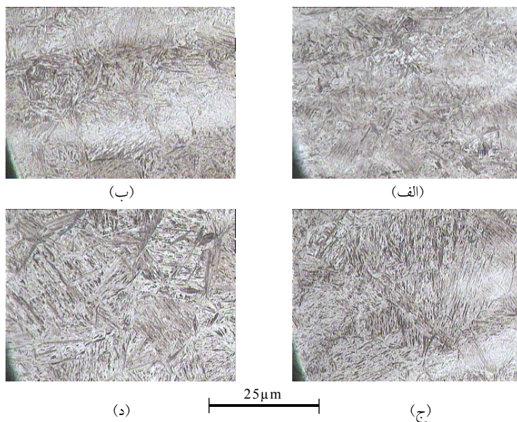
شکل ۹- ریزساختار بینایت ومارتنزیت در آزمایشهای CCCT بعد از اعمال یک مرحله تغییر شکل با \dot{\epsilon} = 0.1 \text{ s}^{-1} و \epsilon = 0.92 در دمای 1100^\circ\text{C} ، در زمانهای مختلف سرد شدن، که با محلول اچ نایتال ۳٪ ریز ساختار بینایت و مارتنزیت در آن ظاهر شده است (الف) 214^\circ\text{C/Sec} (کوئچ)، (ب) 119^\circ\text{C/Sec} (ج) 0.3^\circ\text{C/Sec} (د) 0.2^\circ\text{C/Sec}
