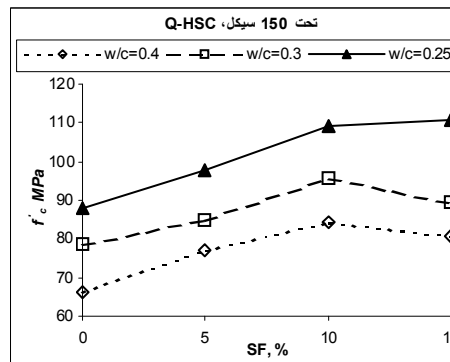
شکل ۹- مقاومت فشاری بتن با درشت دانه کوارتزی در مقابل درصد های میکروسیلیس بعد از ۱۵۰ سیکل
