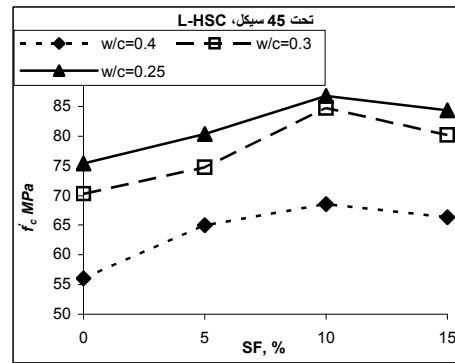
شکل ۱- مقاومت فشاری بتن با درشت دانه آهکی در مقابل درصدهای میکروسیلیس بعد از ۴۵ سیکل
