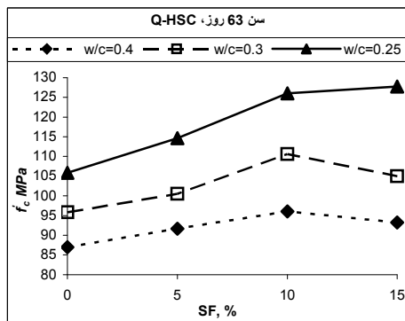
شکل ۱۰- مقاومت فشاری بتن شاهد با درشت دانه کوارتزی در مقابل درصد های میکروسیلیس بعد از ۶۳ روز
