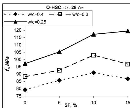
شکل ۸- مقاومت فشاری بتن شاهد با درشت دانه کوارتزی در مقابل درصد های میکروسیلیس بعد از ۲۸ روز
