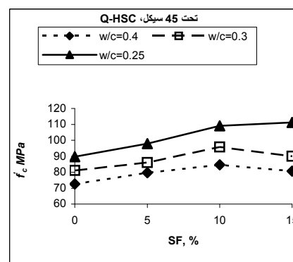
شکل ۷- مقاومت فشاری بتن با درشت دانه کوارتزی در مقابل درصد های میکروسیلیس بعد از ۴۵ سیکل
