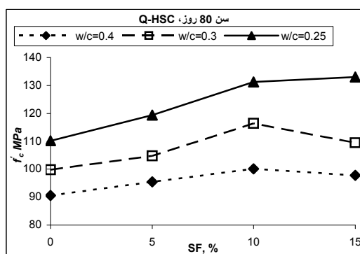
شکل ۱۲- مقاومت فشاری بتن شاهد با درشت دانه کوارتزیتی در مقابل درصدهای میکروسیلیس بعد از ۸۰ روز
