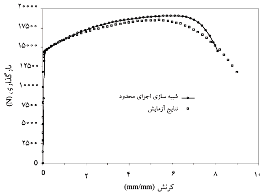
شکل ۹- نمودار "نیرو - جابه جایی در امتداد نیرو" برای نمونه کششی حاصل از آزمون تجربی و شبه سازی اجزای محدود
