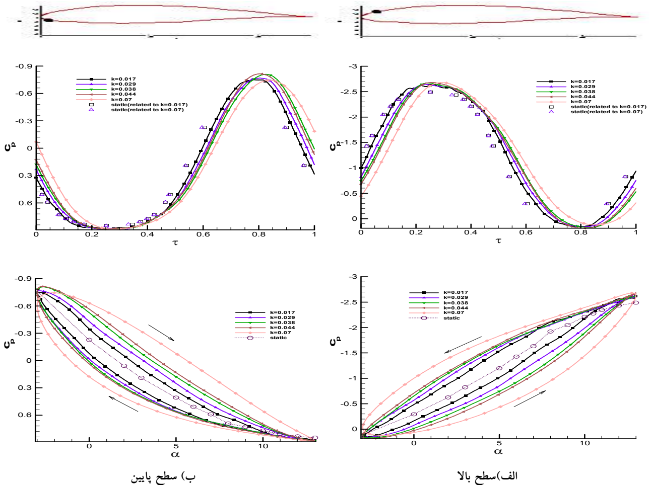
شکل ۱۰-۱ - تاثیر افزایش k در تغییر فشار استاتیکی، x/c = 0.05 ، Re = 0.63 \times 10^6 و \alpha = 5 + 8 \sin(\omega t)
