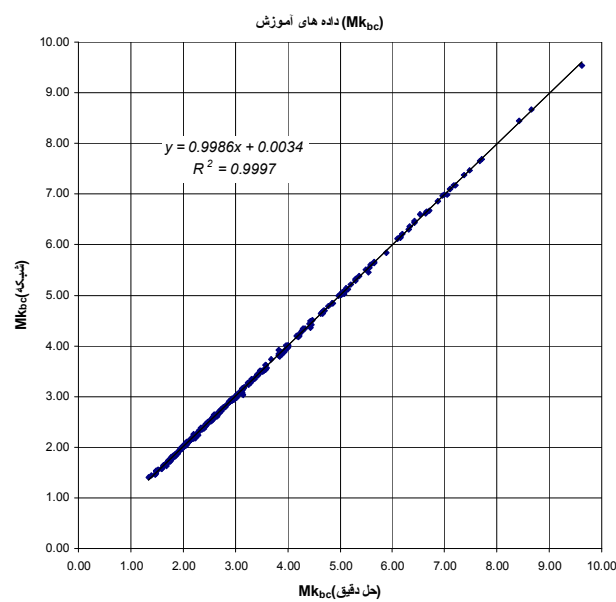
شکل ۱۱- مقادیر Mk_{bc} پیش‌بینی شده توسط شبکه MLP بهینه در برابر مقادیر حل دقیق در دسته داده‌های آموزش
