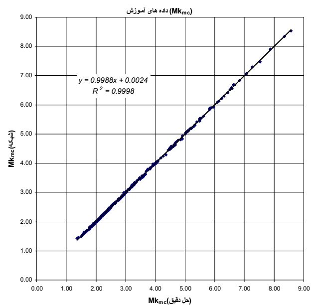
شکل ۱۵- مقادیر Mk_{mc} پیش‌بینی شده توسط شبکه MLP بهینه در برابر مقادیر حل دقیق در دسته داده‌های آموزش
