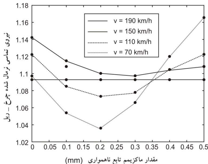
شکل ۱۴- بیشینه نیروی تماسی نرمال شده ریل - چرخ در ریل اصلی (نیروی تماسی استاتیکی نرمال شده) برحسب پارامتر ناهمواری A برای چهار سرعت مختلف وسیله نقلیه (190, 150, 110, 70) در مدل نیم بوژی
