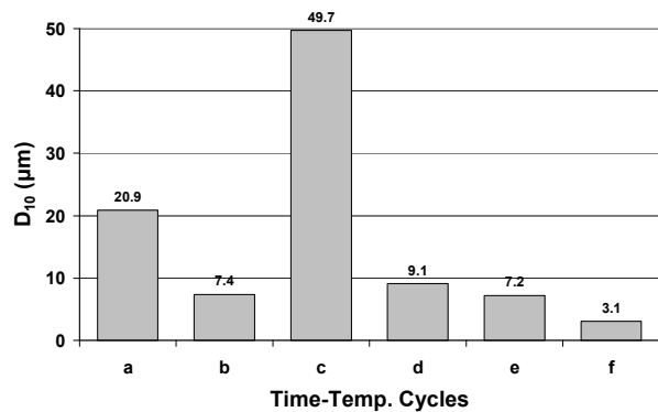
شکل ۴- تاثیر سیکل دما-زمان بر مقدار الف ( D_{10} و ب) ( D_{90} ) پودرها
