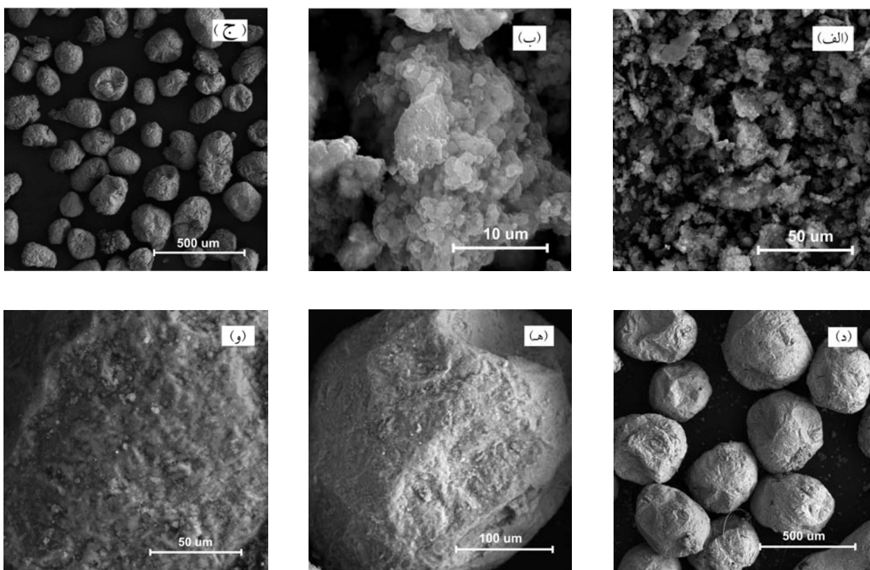
شکل ۱۲- تصاویر SEM ذرات پودر آلیاژ Al-6wt%/Si (الف و ب) در گستره زیر ۳۸ میکرومتر، (ج) ۲۱۲-۱۰۶ میکرومتر و د و ه و (و) ۵۰۰-۳۰۰ میکرومتر تهیه شده توسط سیکل (ه)
