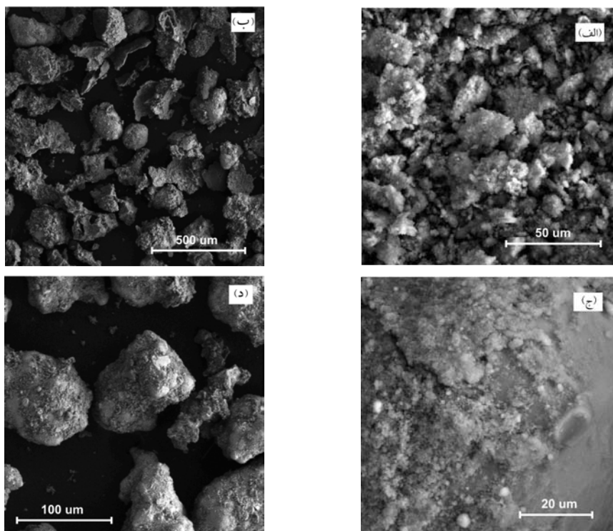
شکل ۱۰- تصاویر SEM ذرات پودر آلیاژ Al-6wt%/Si (الف) در گستره زیر ۳۸ میکرومتر، ب و ج) ۲۱۲-۱۰۶ میکرومتر و (د) ۵۰۰-۳۰۰ میکرومتر تهیه شده توسط سیکل (ج)
