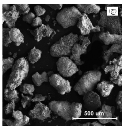
شکل ۹- تصاویر SEM ذرات پودر آلیاژ Al-۶wt%/Si (الف و ب) در گستره زیر ۳۸ میکرومتر، (ج) ۲۱۲-۱۰۶ میکرومتر و (د) ۵۰۰-۳۰۰ میکرومتر تهیه شده توسط سیکل (ب)
