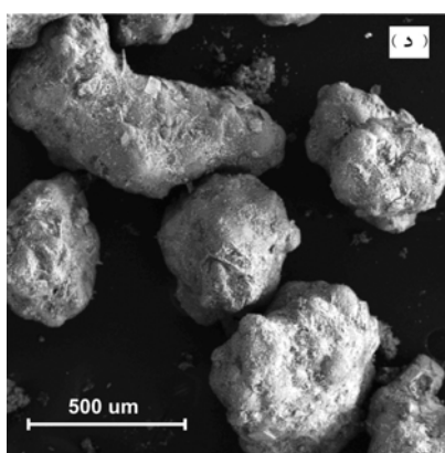
شکل ۹- تصاویر SEM ذرات پودر آلیاژ Al-۶wt%/Si (الف و ب) در گستره زیر ۳۸ میکرومتر، (ج) ۲۱۲-۱۰۶ میکرومتر و (د) ۵۰۰-۳۰۰ میکرومتر تهیه شده توسط سیکل (ب)
