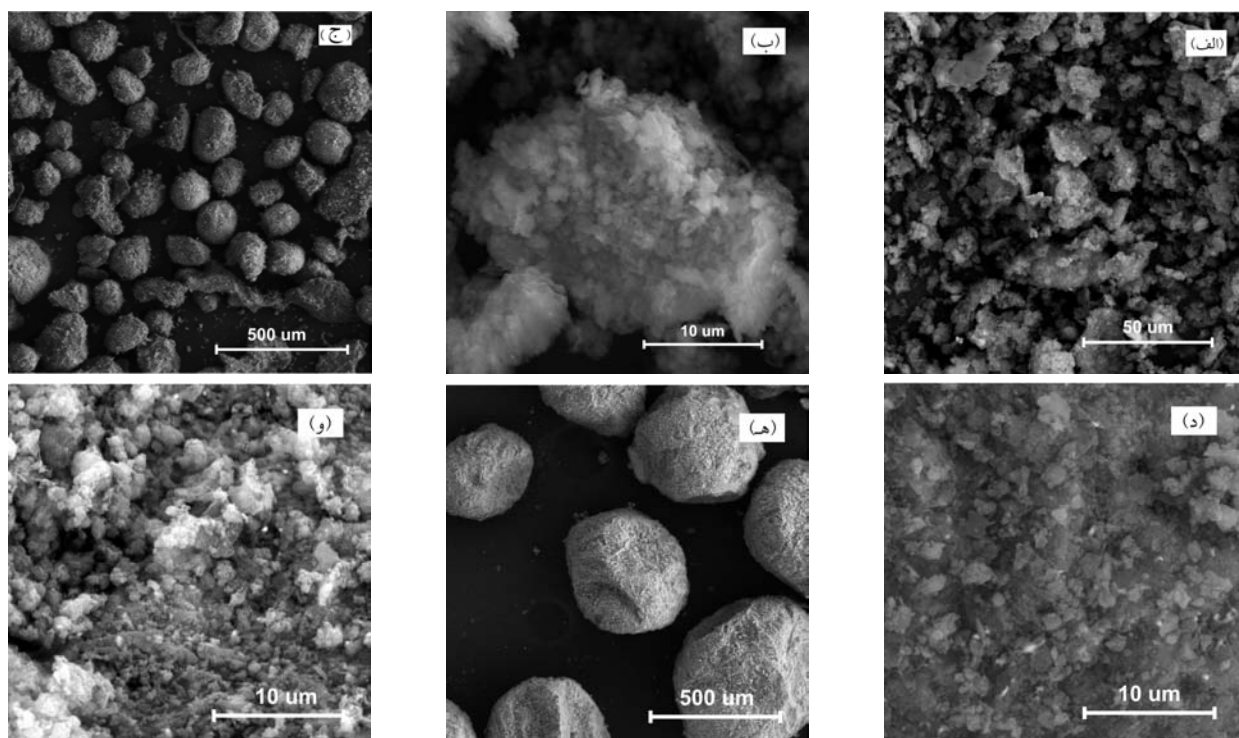
شکل ۱۱- تصاویر SEM ذرات پودر آلیاژ Al-6wt%/Si (الف و ب) در گستره زیر ۳۸ میکرومتر، ج و د) ۲۱۲-۱۰۶ میکرومتر و (ه و و) ۵۰۰-۳۰۰ میکرومتر تهیه شده توسط سیکل (د)
