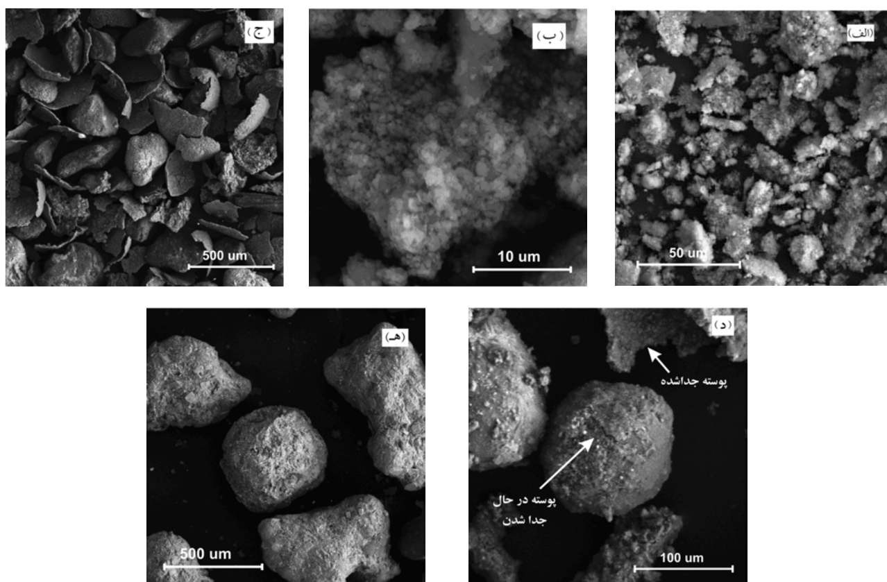
شکل ۸- تصاویر SEM ذرات پودر آلیاژ \text{Al-6wt\%/Si} (الف و ب) در گستره زیر ۳۸ میکرومتر، ج و د) ۲۱۲-۱۰۶ میکرومتر و (ه) ۵۰۰-۳۰۰ میکرومتر تهیه شده توسط سیکل (الف)
