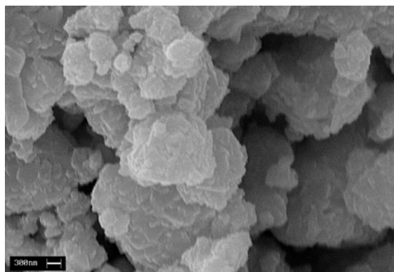
شکل ۷- تصویر SEM زیرکونیای ۸۰ ساعت آسیابکاری شده و سپس آنیل شده در محیط کلر و دمای ۸۰۰°C.
