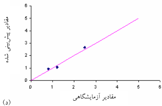
شکل ۳- منحنیهای حاصل از مقادیر پیش بینی شده سرعت سرد شدن (°C/s) توسط شبکه عصبی برحسب مقادیر تجربی
