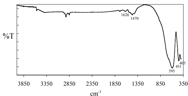
شکل ۲- طیف مادون قرمز تبدیل فوریه برای نمونه تیتانات کلسیم عملیات حرارتی شده در دمای ۸۰۰ درجه سانتیگراد.
