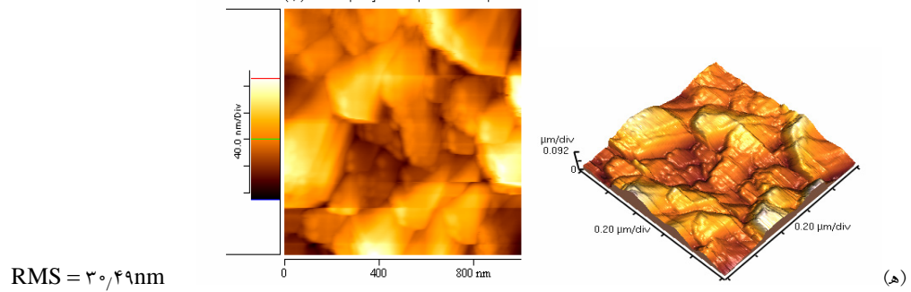
شکل ۲- تصویر میکروسکوپ نیروی اتمی دو بعدی و سه بعدی از سطح تیتانیوم (الف): پولیش شده و اصلاح شده با (ب): ۱۰۰ درصد اسید فلوئوریدریک (ج): ۸۰ درصد اسید کلریدریک- ۶ درصد اسید فلوئوریدریک- ۱۴ درصد اسید فسفریک (د): ۸۵ درصد اسید کلریدریک- ۶ درصد اسید فلوئوریدریک- ۹ درصد اسید فسفریک (ه): ۸۰ درصد اسید کلریدریک- ۱۰ درصد اسید فلوئوریدریک- ۱۰ درصد اسید فسفریک، به مدت ۱۲۰ ثانیه و در دمای محیط.
