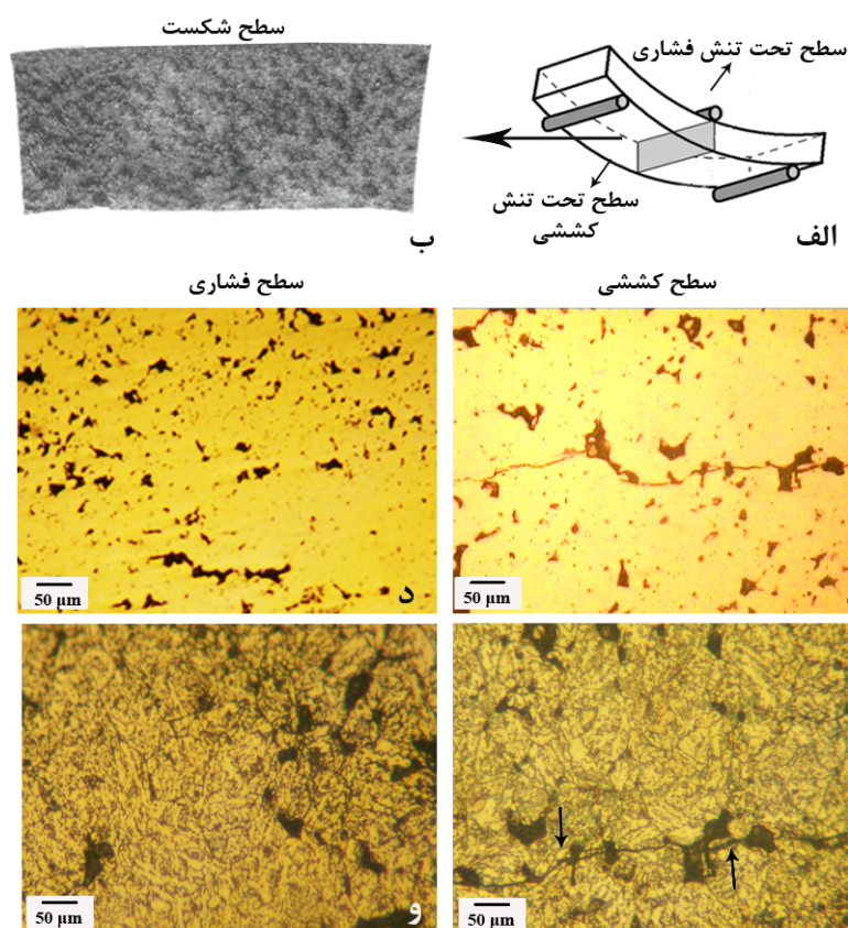
شکل ۶- الف) شماتیک نحوه اعمال بارهای کششی و فشاری که به سطوح نمونه وارد می‌شوند، ب) تصویر ماکرو سطح شکست از نمونه، ج) سطح تحت تنش کششی با حضور ترک (پیکانها)، د) سطح تحت فشار که ترکی در آن مشاهده نمی‌شود، ه) سطح اچ شده شکل ج که نشان می‌دهد مسیر ترک از میان مناطق بینیتی/مارتنزیتی و تخلخلها است و و) سطح اچ شده شکل د.
