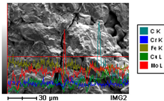
شکل ۸- الف) تصویر SEM-Map از رشد ترک در سطح تحت کشش و ب) تحلیل EDS از این منطقه.
