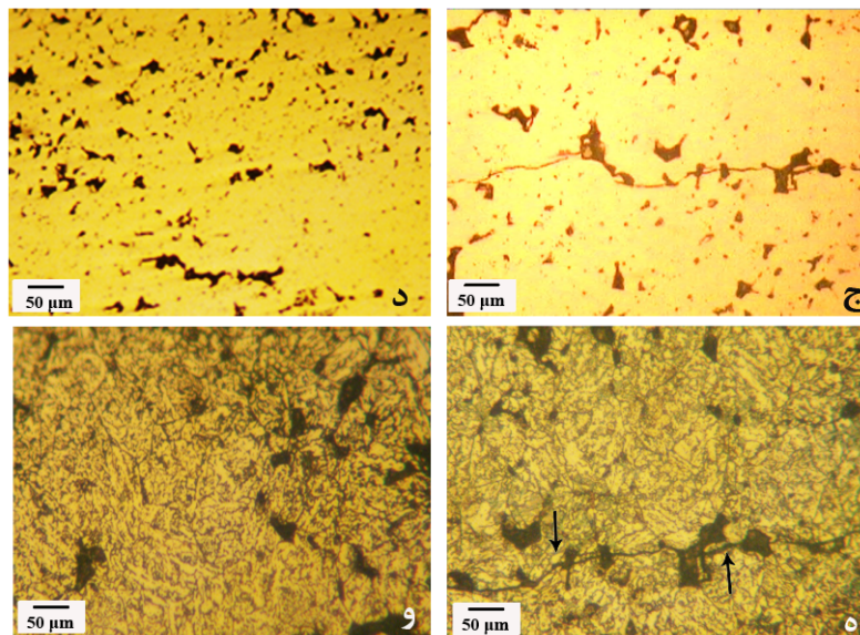
شکل ۶- الف) شماتیک نحوه اعمال بارهای کششی و فشاری که به سطوح نمونه وارد می‌شوند، ب) تصویر ماکرو سطح شکست از نمونه، ج) سطح تحت تنش کششی با حضور ترک (پیکانها)، د) سطح تحت فشار که ترکی در آن مشاهده نمی‌شود، ه) سطح اچ شده شکل ج که نشان می‌دهد مسیر ترک از میان مناطق بینیتی/مارتنزیتی و تخلخلها است و و) سطح اچ شده شکل د.
