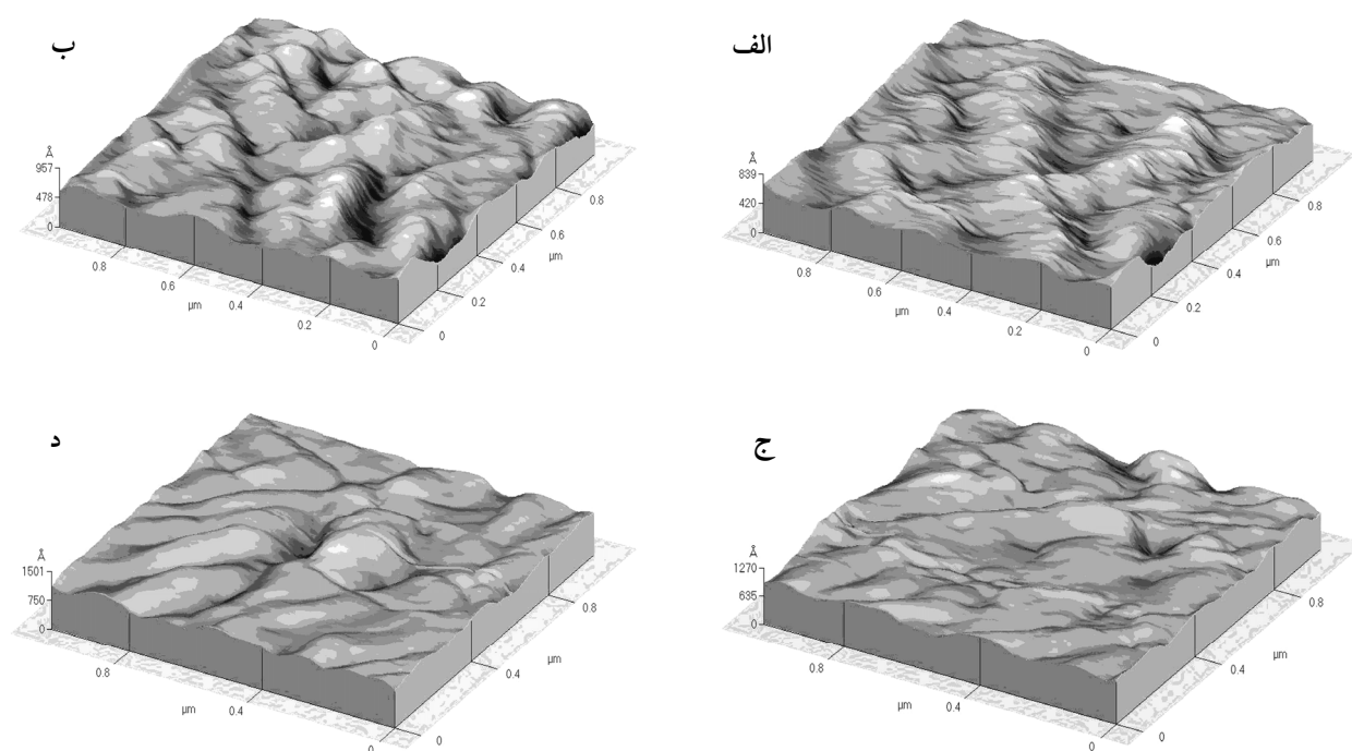
شکل ۱- تصاویر میکروسکوپ نیروی اتمی سه بعدی از نانوکامپوزیتهای پلی استر- سیلیس تهیه شده: الف) پلی استر خالص، ب) نانوکامپوزیت پلی استر- ۵٪ نانوسیلیس آبدوست ۱، ج) نانوکامپوزیت پلی استر- ۵٪ نانوسیلیس آبدوست ۲، د) نانوکامپوزیت پلی استر- ۵٪ نانوسیلیس آبریز
