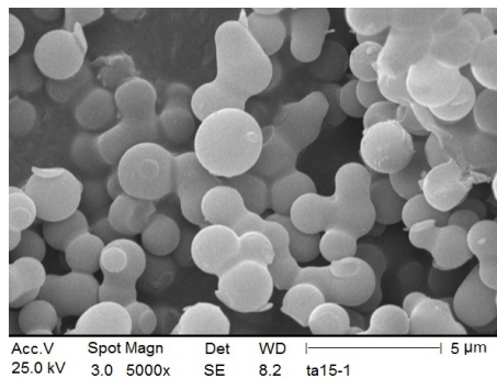
شکل ۶- نمونه سنتز شده به همراه ۰/۱۸ گرم لانتانیم و ۳۰ دقیقه امواج اولتراسونیک
