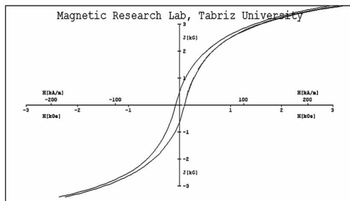
شکل ۲- (الف) فریت باریم آلیایده نشده [۸] (ب) فریت باریم آلیایده شده با Mn و Zr
