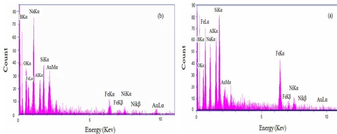
شکل ۶- آنالیز EDS مربوط به (a) بلورهای مکعبی و (b) بلورهای میله‌ای.
