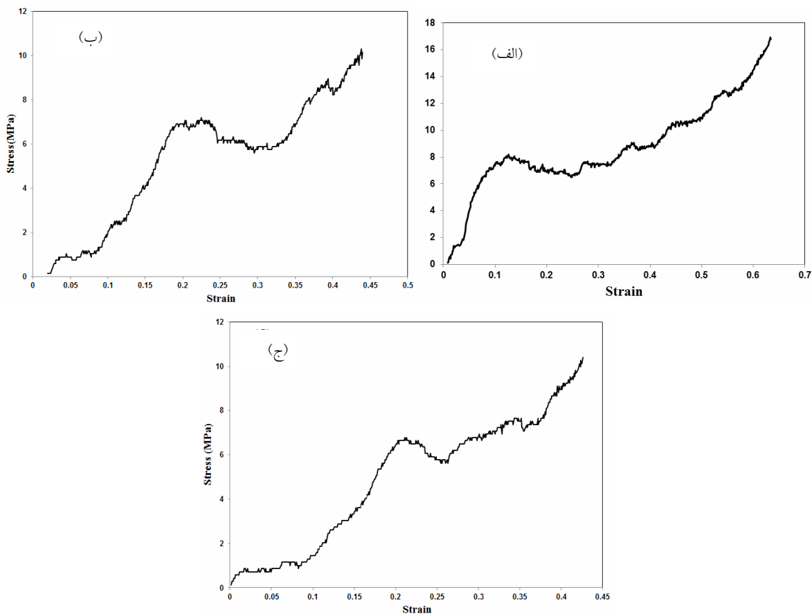
شکل ۲- نمودار تنش - کرنش سه نوع داربست (الف) ۲۰/۸۰، (ب) ۷۰/۳۰ و (ج) ۴۰/۶۰.
