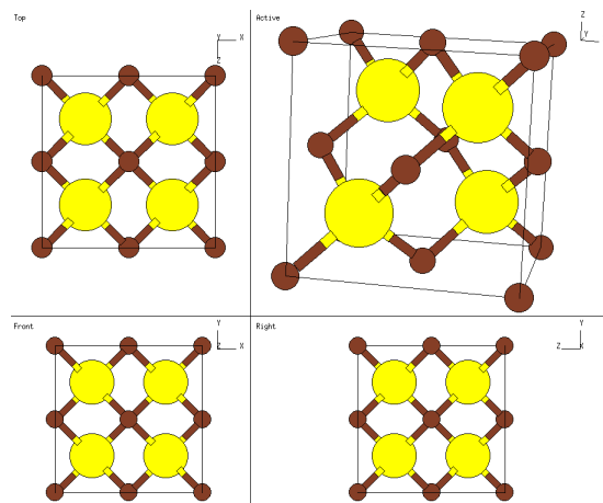
شکل ۲- ساختار بلوری سیلیکون کاربرد 3C-SiC (β) از منظرهای مختلف (گلوله‌های قهوه ای اتم‌های سیلیکون و گلوله‌های زرد اتم‌های کربن هستند)
