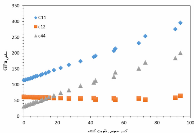
شکل ۶- پیش‌بینی ثوابت ماتریس سفتی با استفاده از شبیه‌سازی دینامیک مولکولی در برابر تغییرات کسر حجمی تقویت‌کننده SiC
