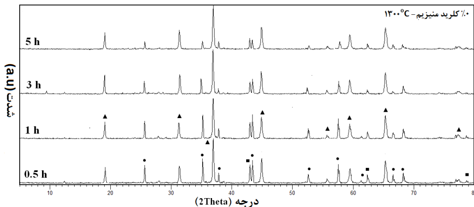
شکل ۱- نتایج تحلیل فازی ترکیبات بدون افزودنی کلرید منیزیم پخته شده در دمای ۱۳۰۰°C و در زمان‌های مختلف ■: Periclase, ▲: Spinel, ●: Corundum
