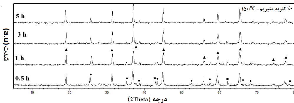
شکل ۴- نتایج تحلیل فازی ترکیبات بدون افزودنی پخته شده در دمای ۱۵۰۰°C و در زمان‌های مختلف
