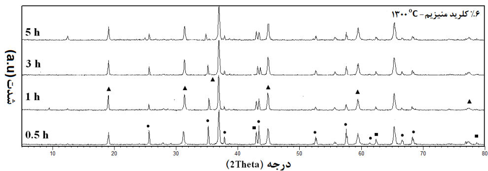
شکل ۲- نتایج تحلیل فازی ترکیبات حاوی ۶ درصد کلرید منیزیم پخته شده در دمای ۱۳۰۰°C و در زمان‌های مختلف
