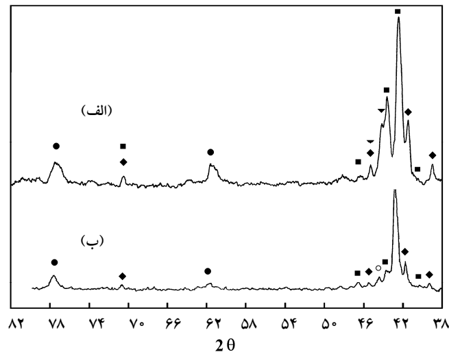
شکل ۱۰- الگوی پراش اشعه ایکس (الف) نمونه سنتز احتراقی و (ب) نمونه تفجوشی شده علائم در شکل نشان دهنده \bullet NiTi، \blacklozenge \text{Ni}_2\text{Ti} ، \blacksquare \text{Ni}_3\text{Ti} ، \blacktriangledown \text{Ni}_{0.67}\text{Ti}_{0.33} و \circ Ni هستند.
