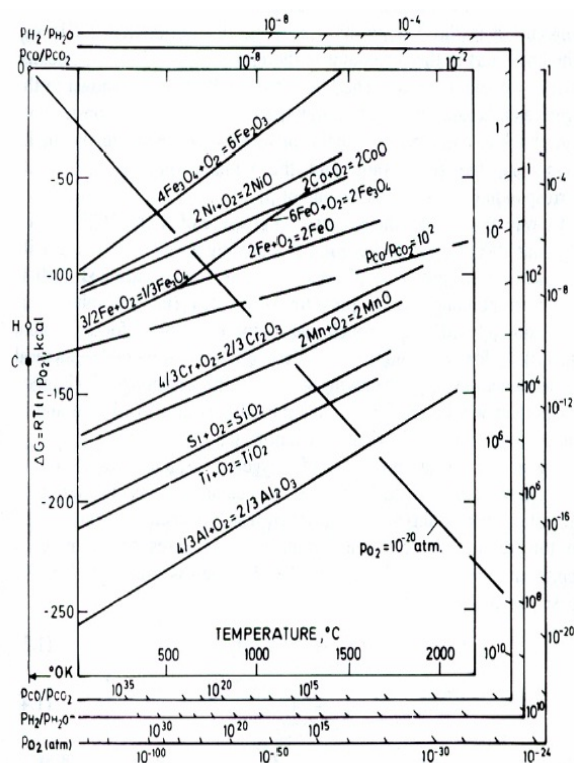
شکل ۳- دیاگرام الینگهام [۲۱].
