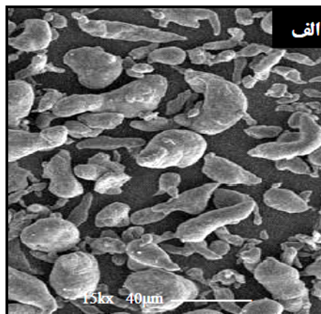
شکل ۱- تصویر میکروسکوپ الکترونی روبشی (SEM): الف) پودر آلومینیوم و ب) پودر دی اکسید تیتانیم.
