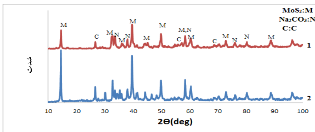
شکل ۳- الگوی پراش پرتو ایکس مخلوط پودری مولیبدنیت، گرافیت، کربنات سدیم (۱: بدون حرارت دهی و ۲: حرارت دهی تا دمای ۴۰۰ درجه سانتی گراد)
