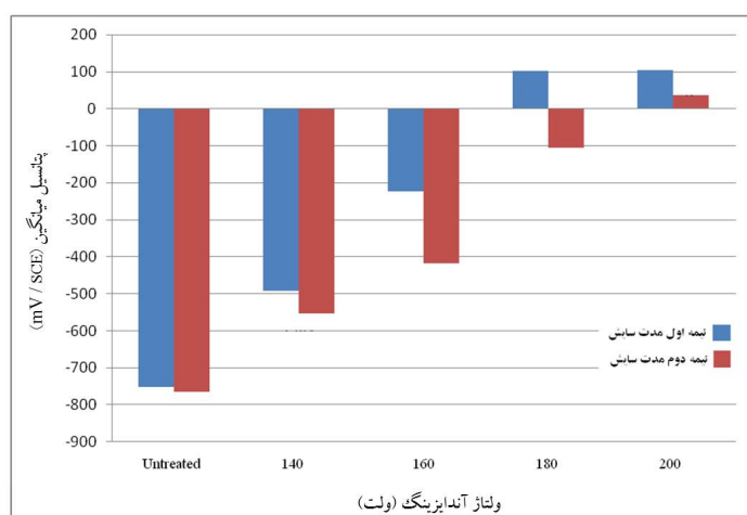
شکل ۶ - مقادیر میانگین پتانسیل در نیمه اول و دوم مدت زمان سایش برای نمونه خام و نمونه‌های آندایز شده در ولتاژهای مختلف.
