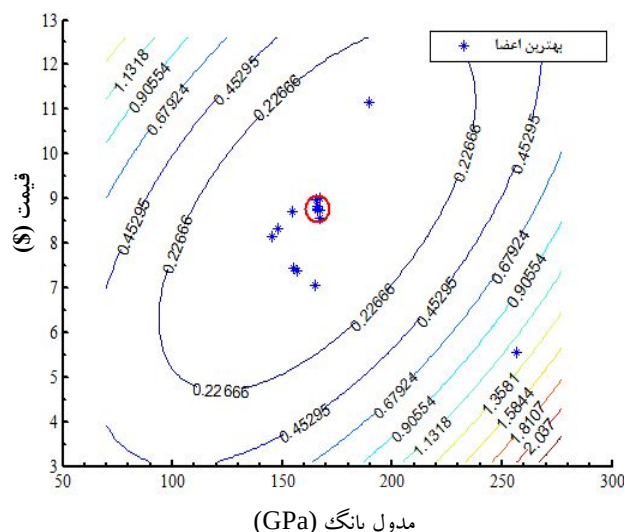
شکل ۴- بهترین اعضای هر نسل در صفحه مدول یانگ و قیمت
